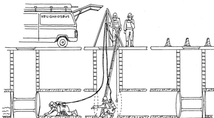
Figuur 4 Betreding bij 3-putsinrichting, waarbij de meting heeft uitgewezen dat dragen van de beademingsapparatuur noodzakelijk is. De personen die afgedaald zijn, dienen aangelijnd te zijn.
