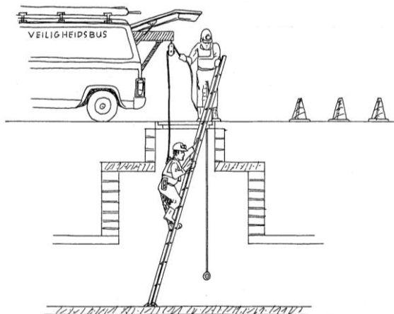
Figuur 1 Afdaling in standaardwerkplekinrichting waarbij de meting aangeeft dat betreding van de put mogelijk is
