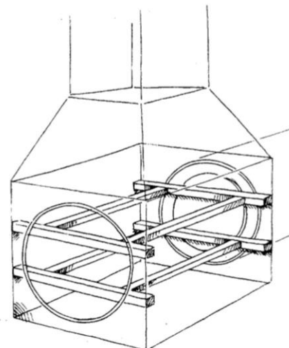
Figuur 5 Voorbeeld van stempelen Rioolafsluitingen moeten zo worden aangebracht dat verwijderen veilig van buiten riool/besloten ruimte mogelijk is
