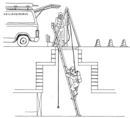
Figuur 2 Afdaling in 1-putsinrichting, waarbij meting aangeeft dat dragen van beademingsapparatuur nodig is
