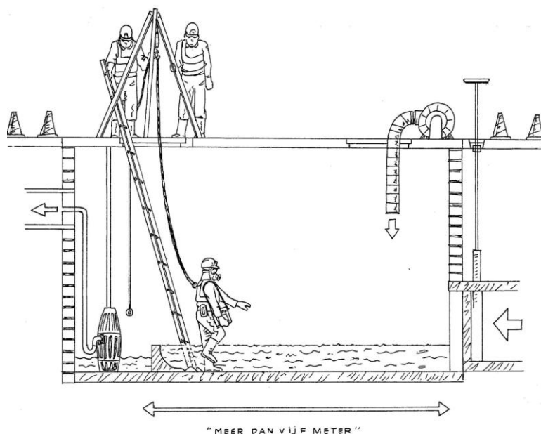
Figuur 3 Afdaling in 2-putsinrichting, waarbij meting aangeeft dat dragen van beademingsapparatuur nodig is.
