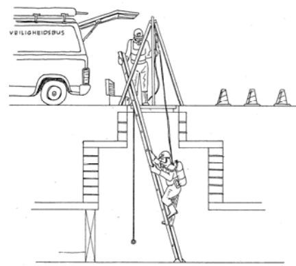
Figuur 2 Afdaling in 1-putsinrichting, waarbij meting aangeeft dat dragen van beademingsapparaat nodig is
